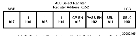
ALS Select Register (2-ALS Version Only) Internal Hex Address: 0x52
