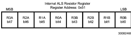
ALS Resistor Control Register Description Internal Hex Address: 0x51
